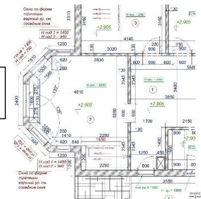
Uyni chizish Чертеж дома
